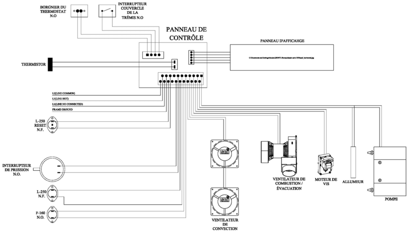
Figure 52 Diagramme électrique
