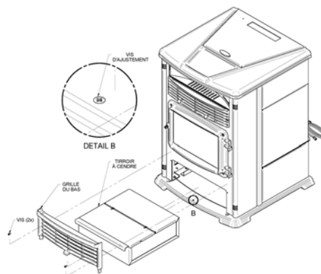
Figure 45 Tiroir à cendre
