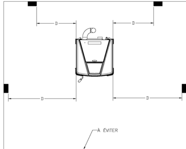
Figure 41 Positionnement du thermostat
