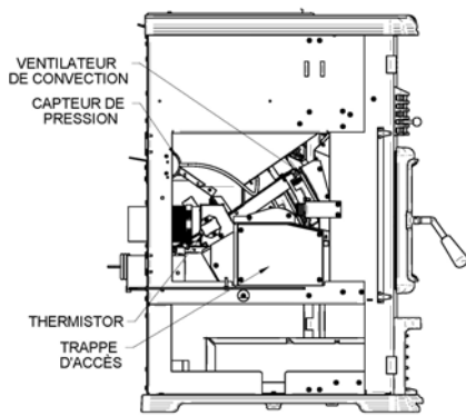
Figure 53 Composantes côté gauche
