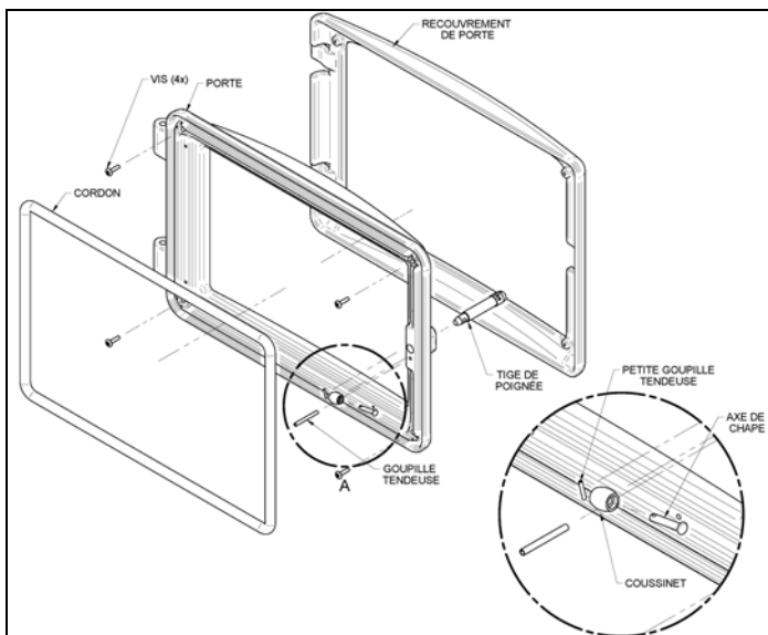
Figure 36 Installation du revêtement de porte
