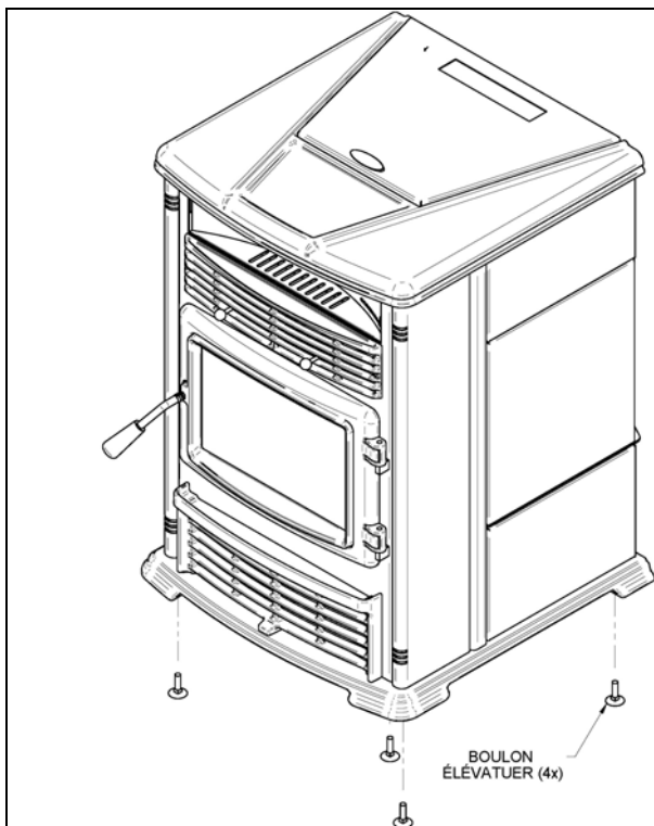
Figure 37 Nivelage de l'appareil
