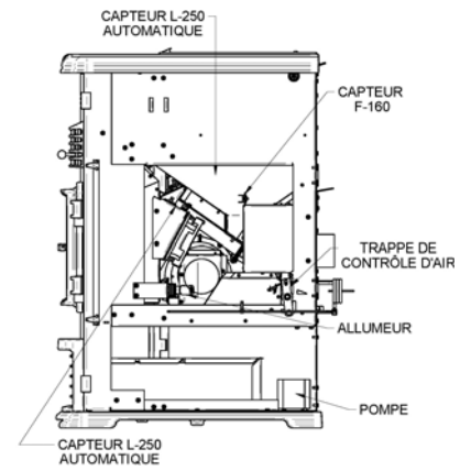
Figure 55 Composantes côté droit
