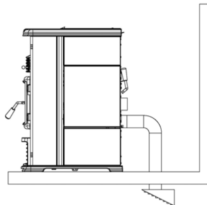
Figure 6 Apport d'air frais d'un vide sanitaire ventilé
