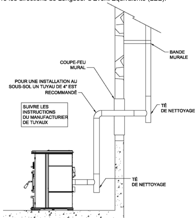
Figure 17 Installation au sous-sol
